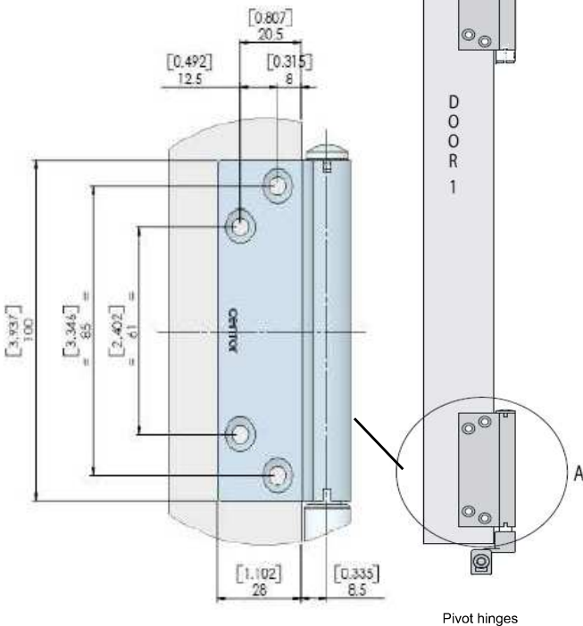
Pivot hinges
