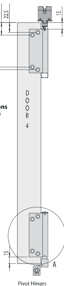
Pivot Hinges
