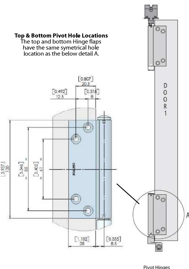
Pivot Hinges
