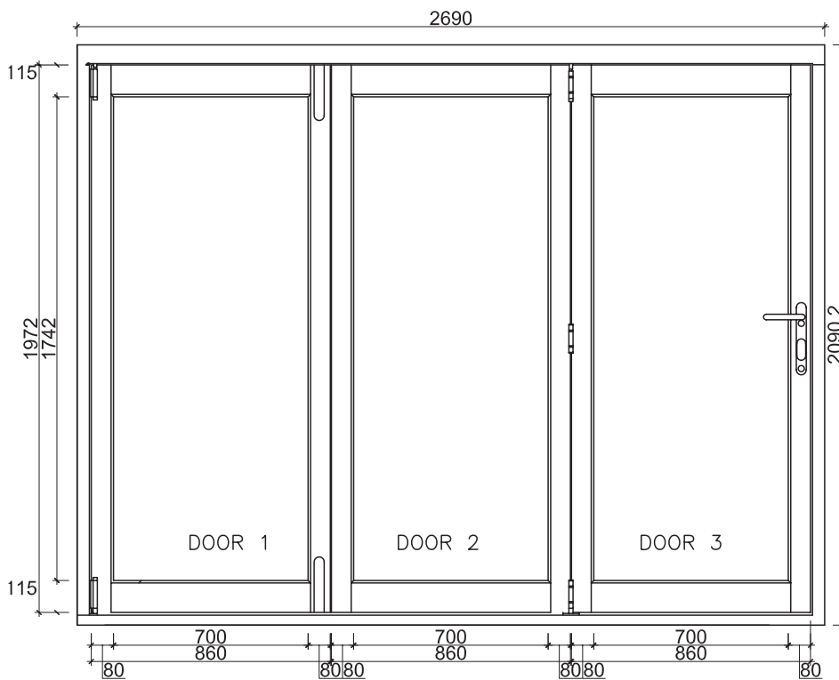
DOOR DIMENSIONS
