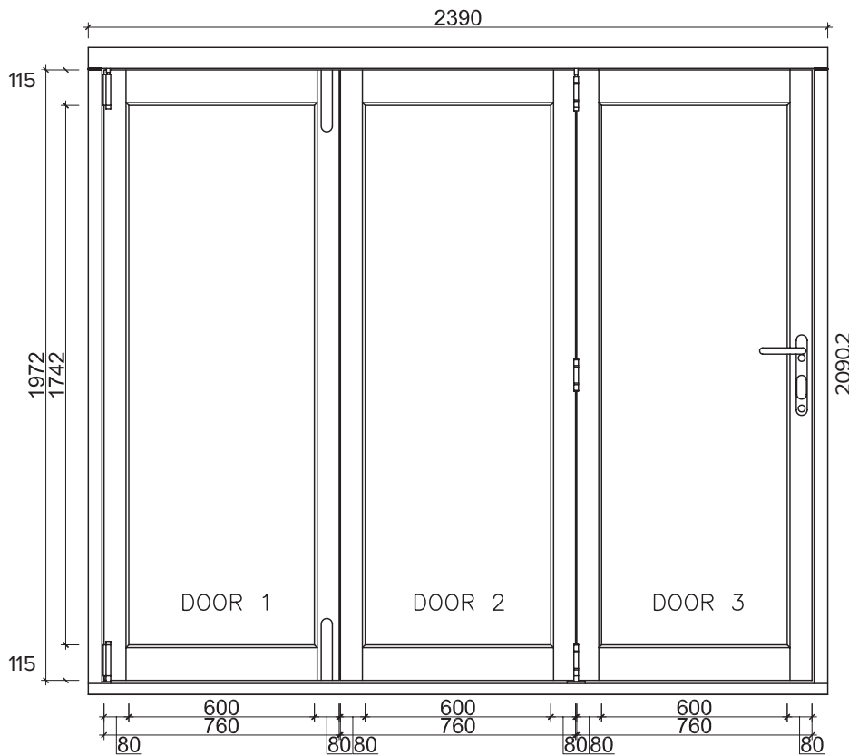
DOOR DIMENSIONS
